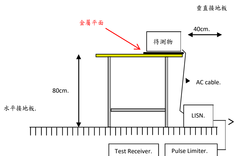
圖一：明緯 EMI 測試系統配置圖
